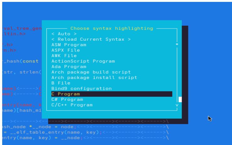
Рисунок 34: Цветовыделение синтаксиса
