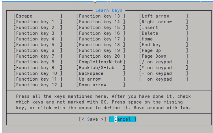
Рисунок 25: Распознавание клавиш
