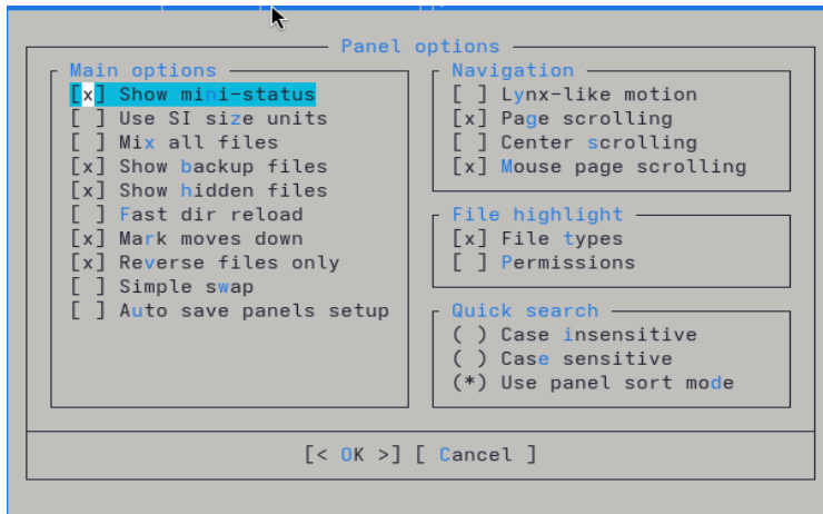
Рисунок 21: Настройки панелей
