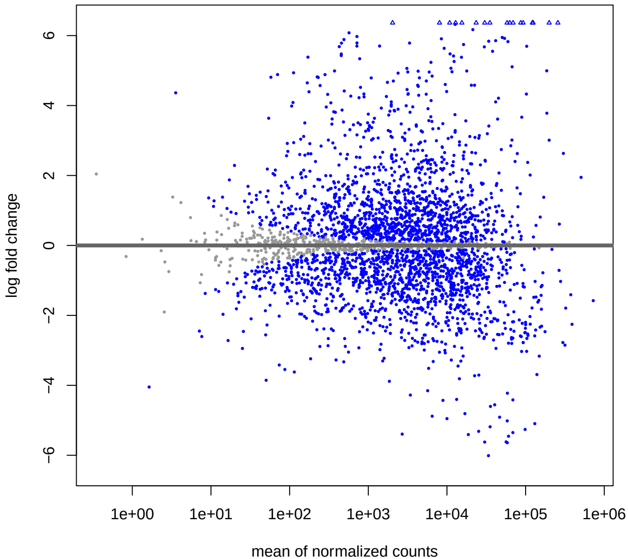
DESeq2 MA Plot
