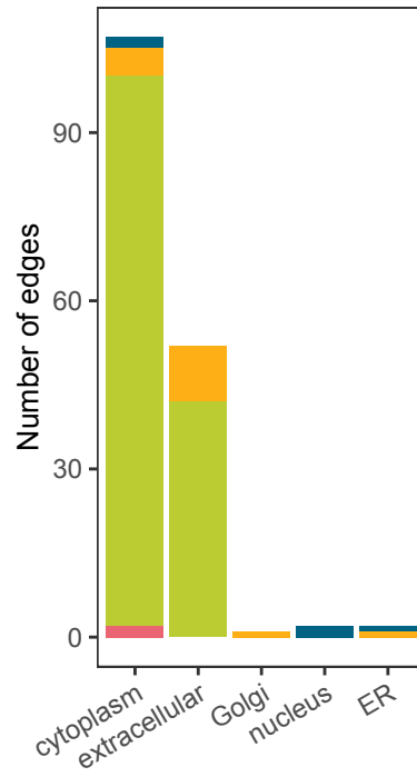
EGFR up
