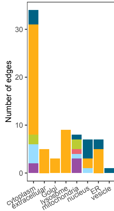
EGFR down
