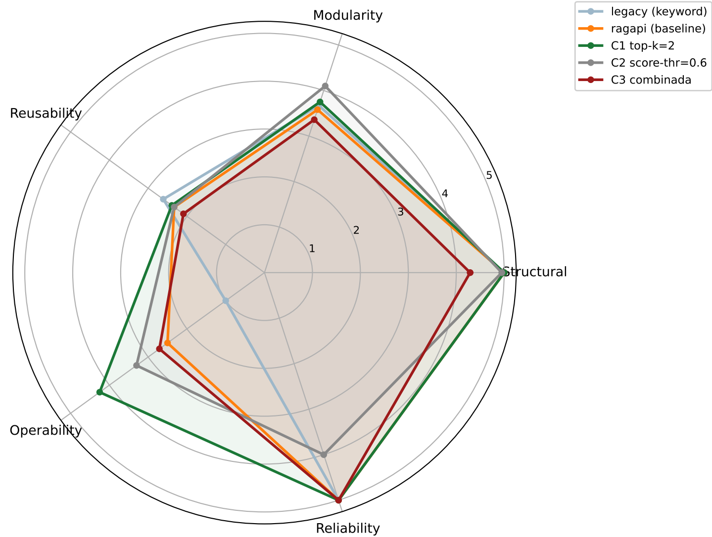
B) Sub-características OQuaRE por configuración
