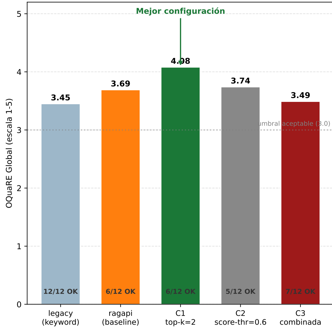
A) Calibración del RAG para Llama 3.1 8B en E3 Global y nº de runs válidas por configuración
