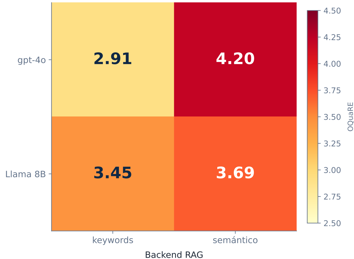
B) Cuadro 2×2 OQuaRE Global
