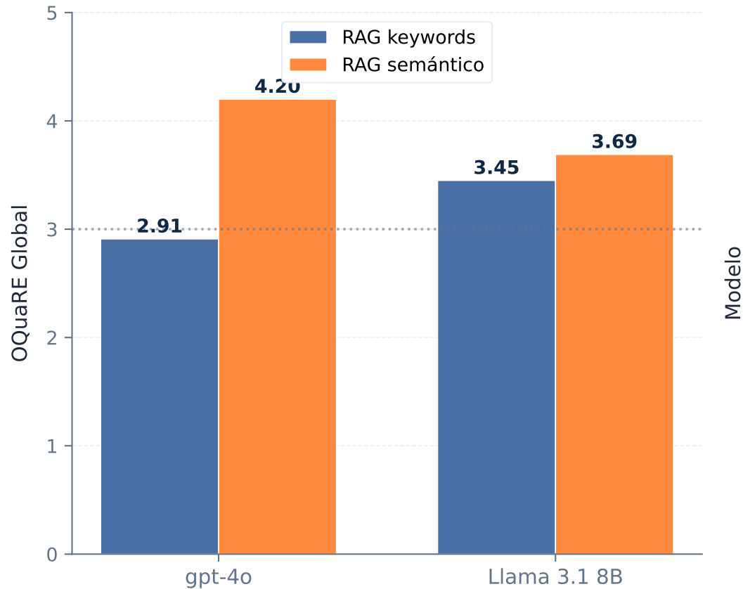
A) Efecto del backend RAG por modelo
