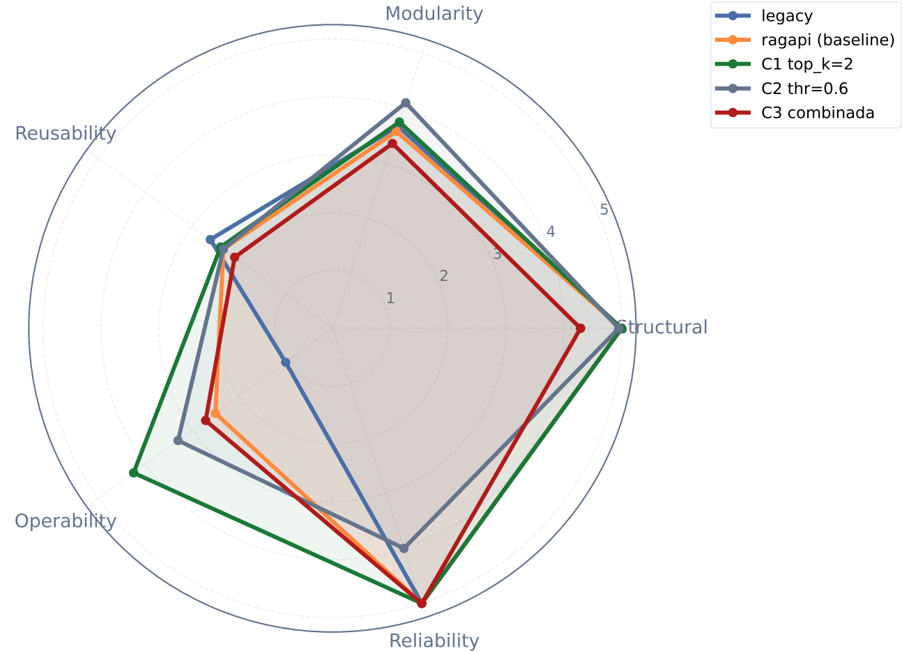
B) Sub-características OQuaRE por configuración
