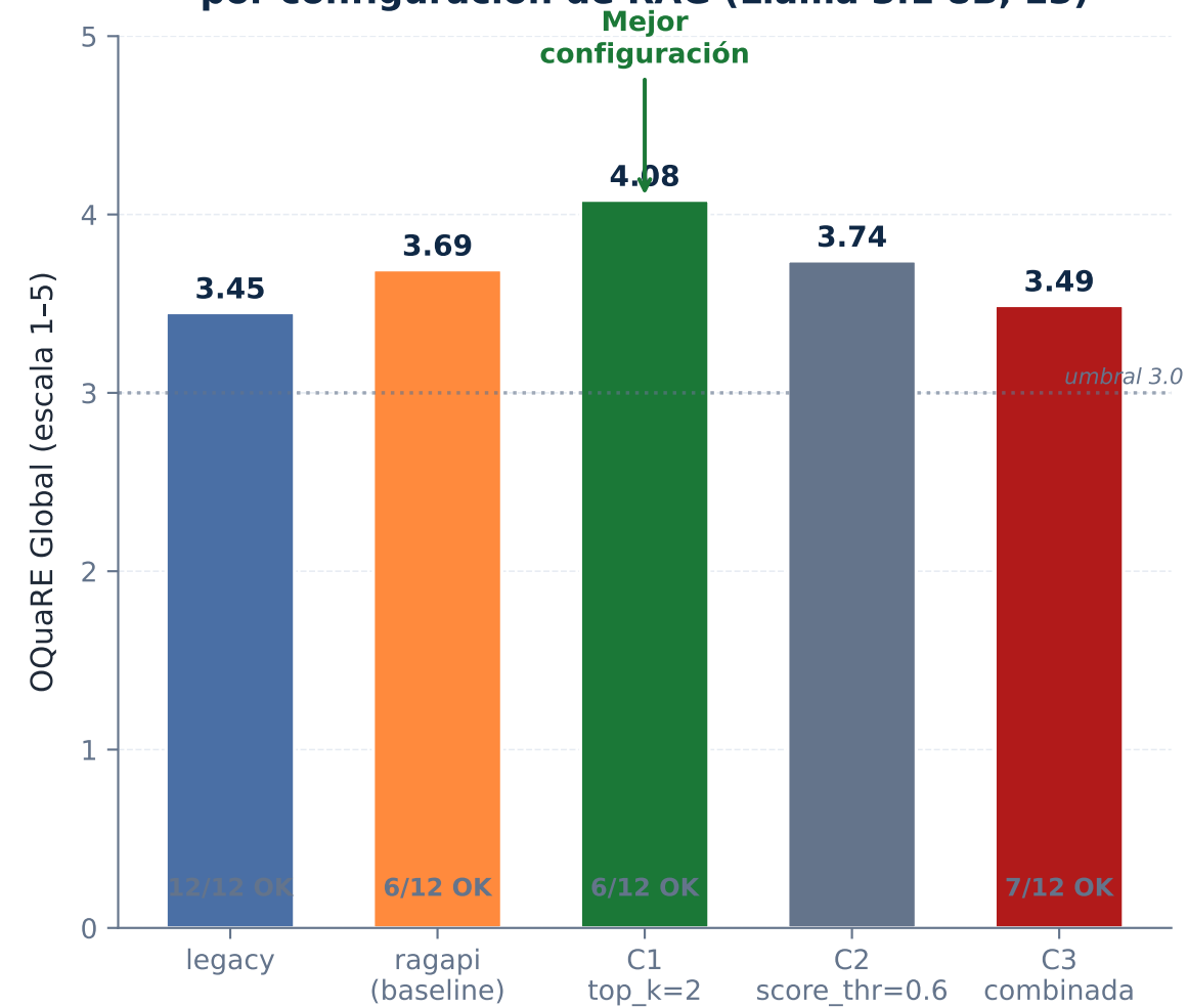
A) OQuaRE Global y nº de corridas válidas por configuración de RAG (Llama 3.1 8B, E3)
