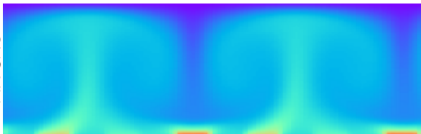
MA-SAC
