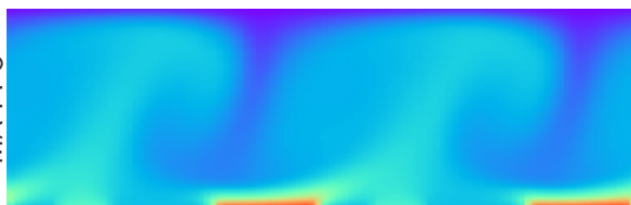
MA-PPO
