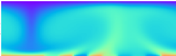
SAC
