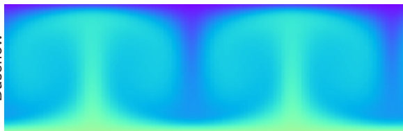
Easy
