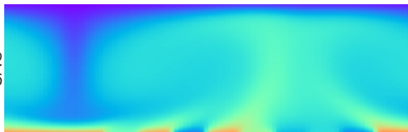
SAC
