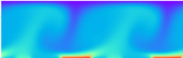
MA-PPO
