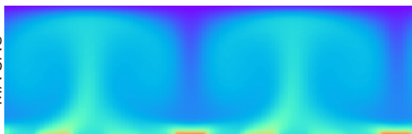
MA-SAC
