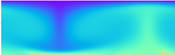
PPO
