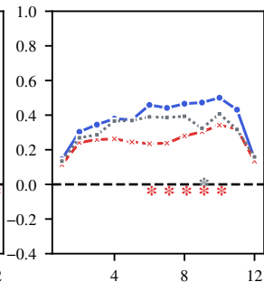
RoBERTa
