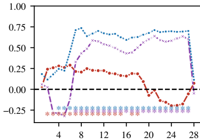
Layer
