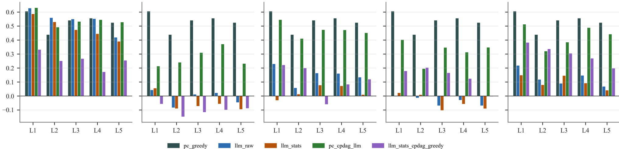
GPT-5.5
