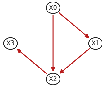
LLM output
