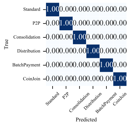
BERT4ETH
