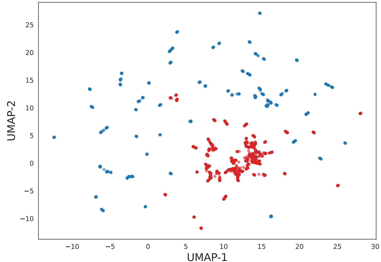
UMAP 2D
