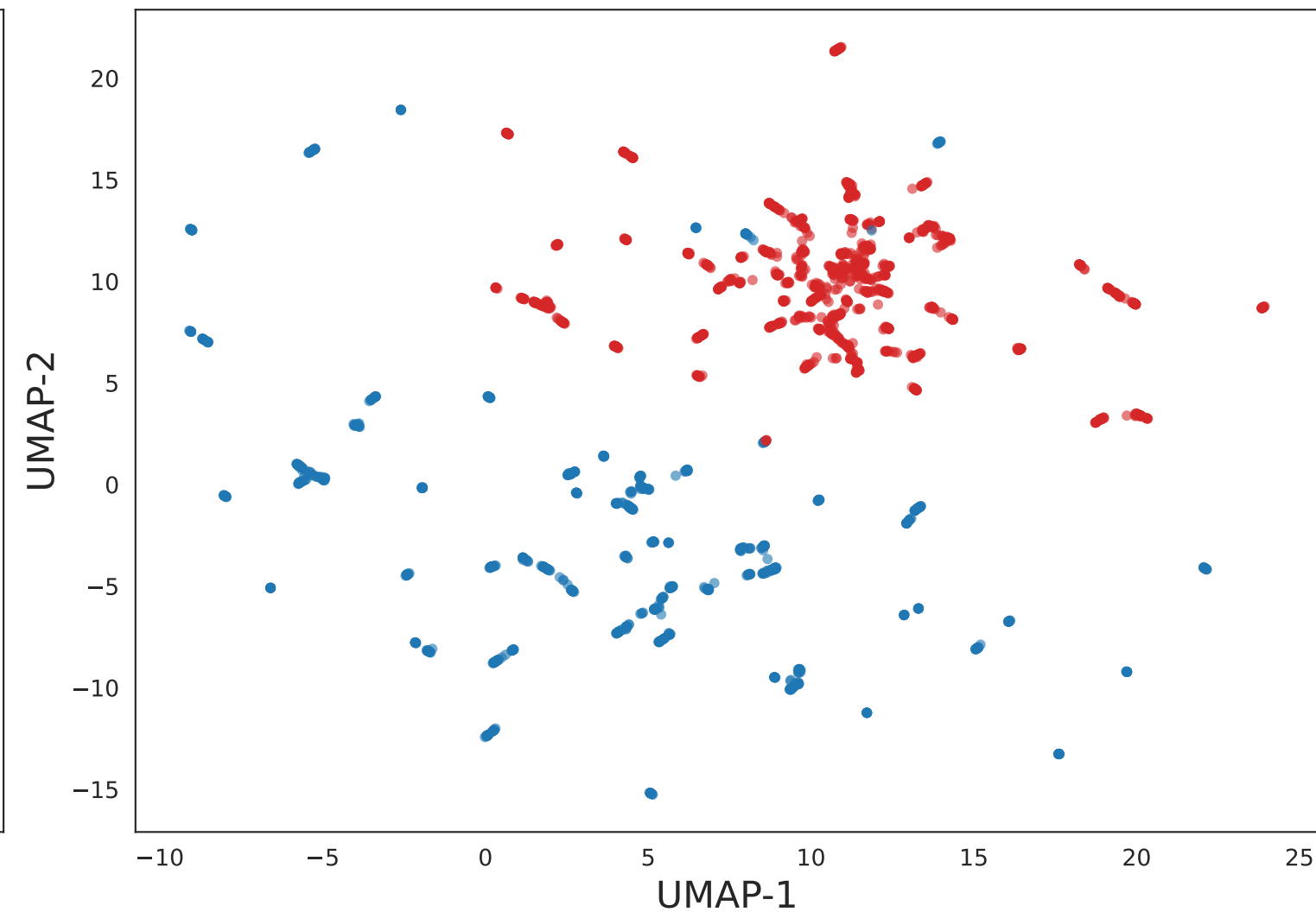
UMAP 2D
