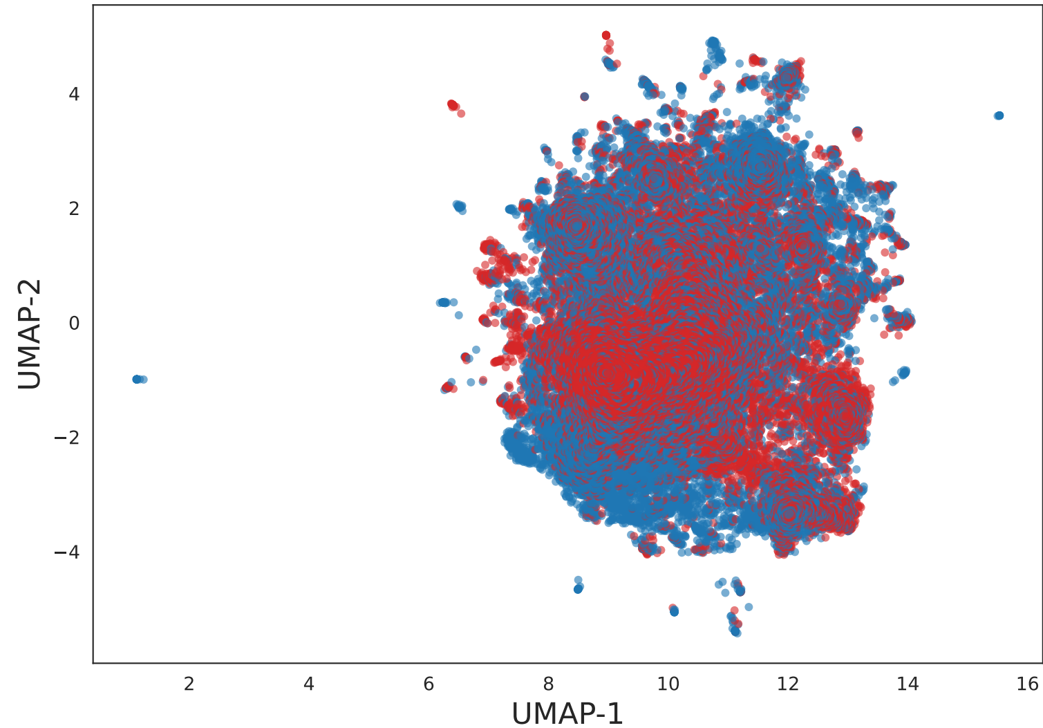
UMAP 2D
