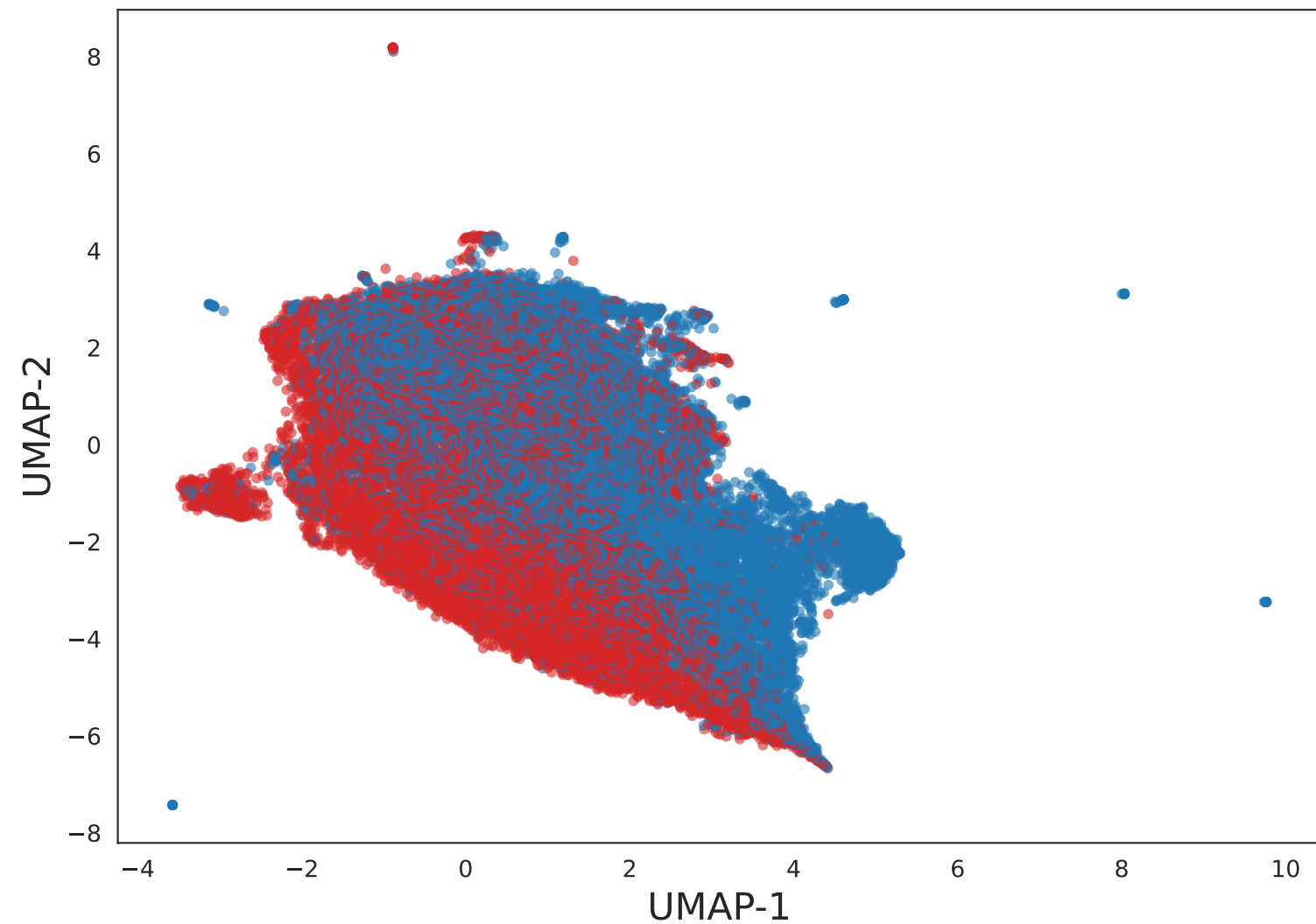
UMAP 2D
