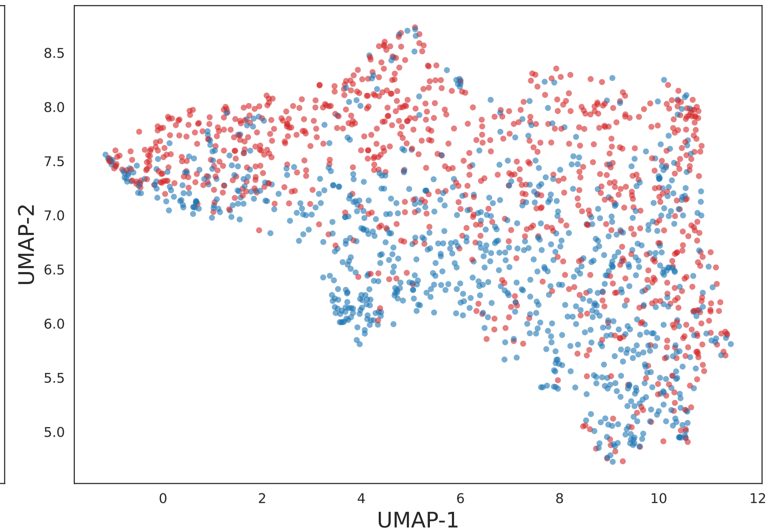
UMAP 2D
