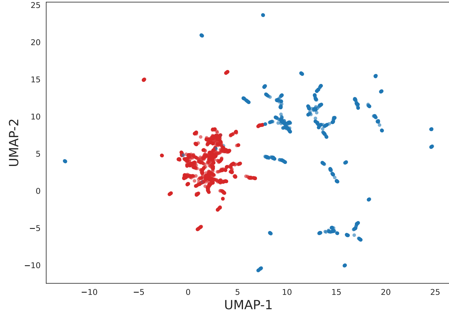
UMAP 2D
