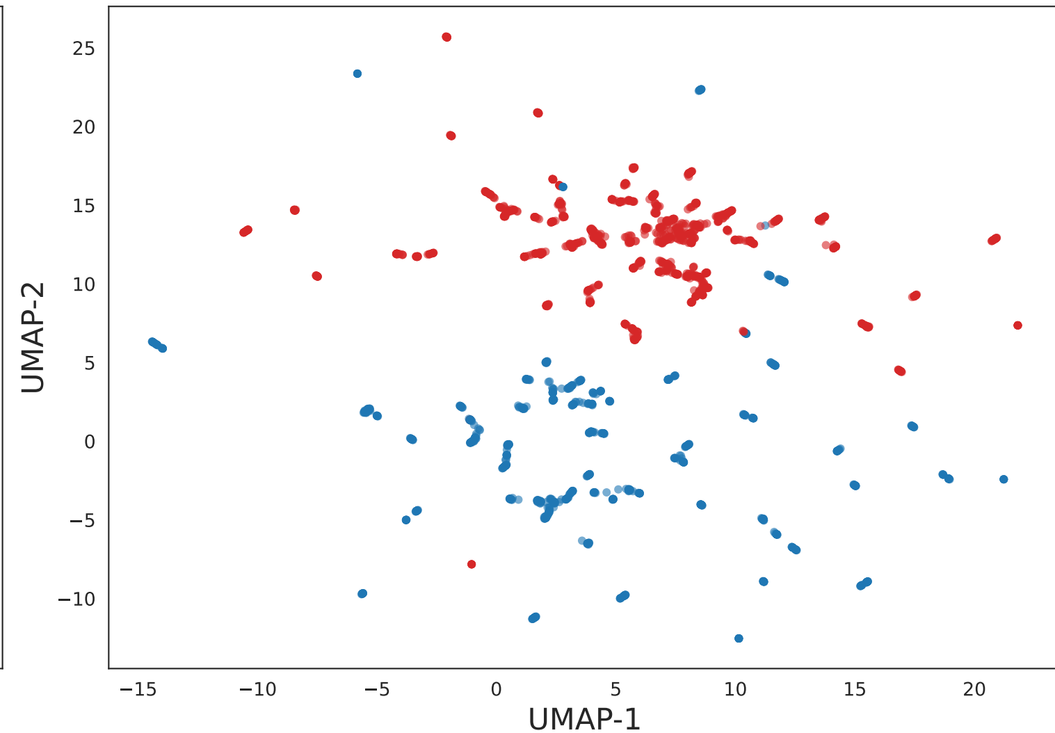
UMAP 2D
