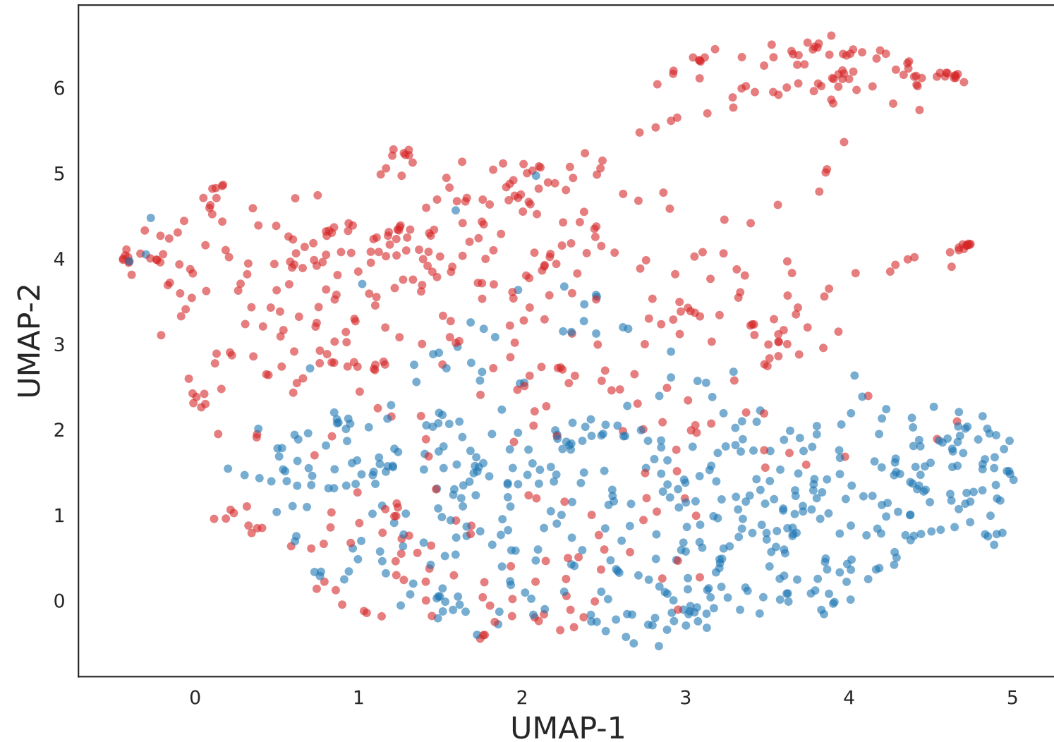
UMAP 2D
