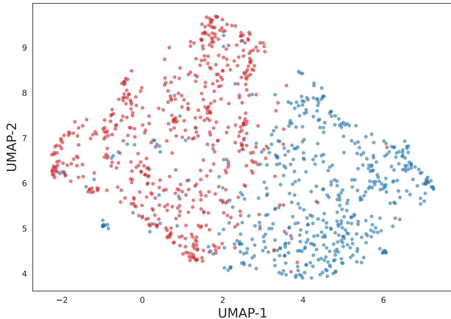
UMAP 2D
