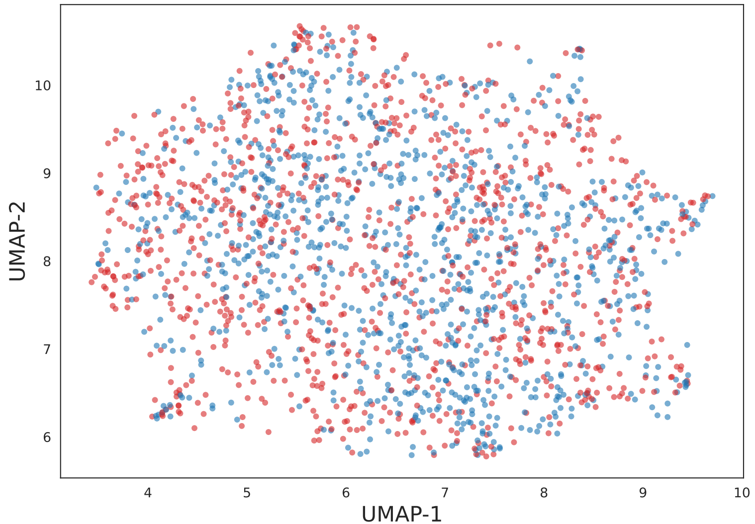
UMAP 2D
