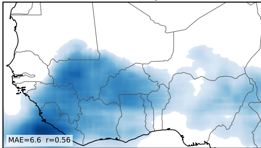
U-Net-Simple
