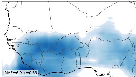
U-Net-SE
