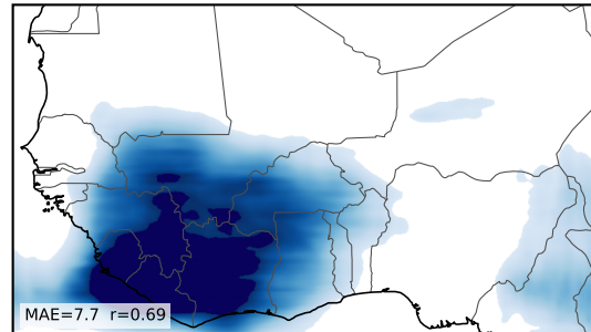
U-Net-CBAM + QM
