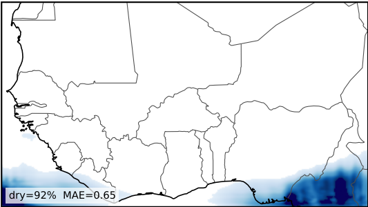
U-Net-CBAM + QM
