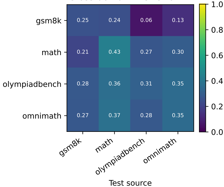
Cross-domain first-error F1
