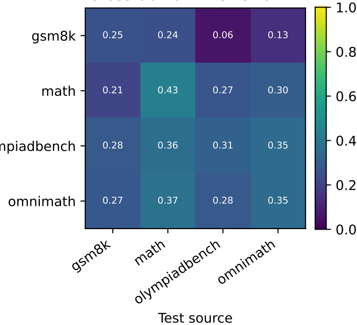
Cross-domain first-error F1
