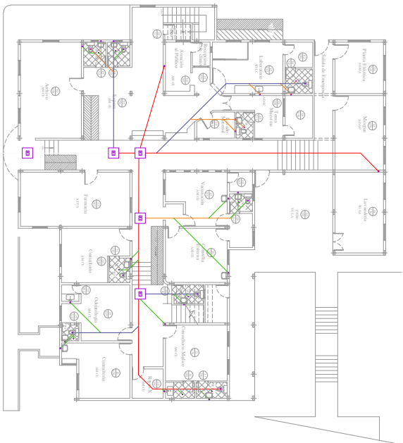
PLANTA DESA/DES PRIMER NIVEL Escala 1:100
