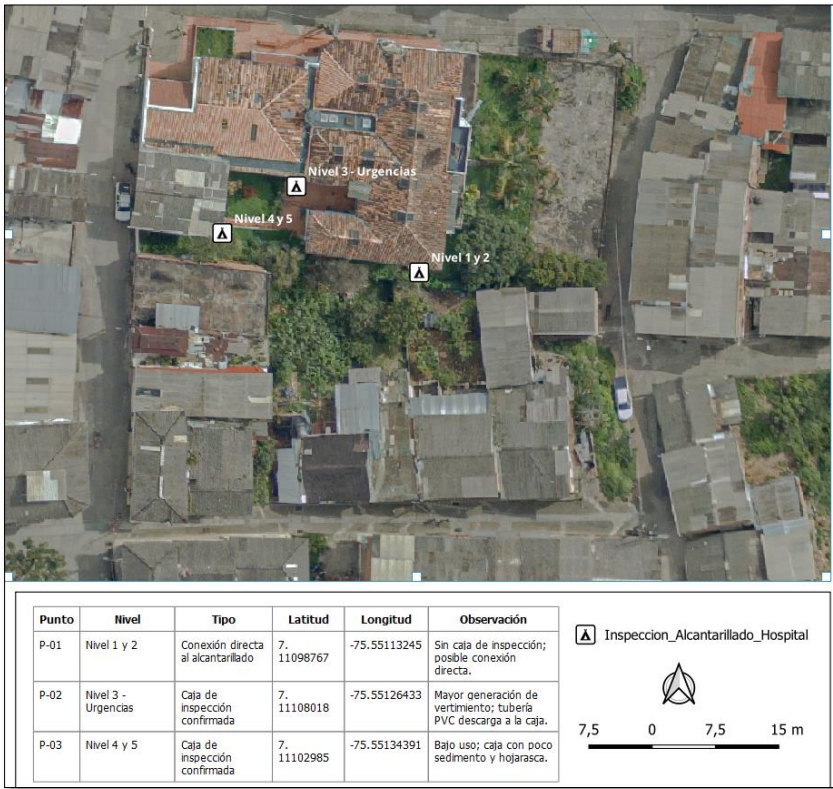
Mapa de puntos de verificación del sistema de alcantarillado – ESE Hospital El Sagrado Corazón, Briceño
