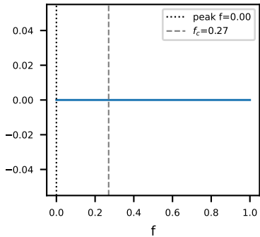
ER \langle k \rangle = 4
