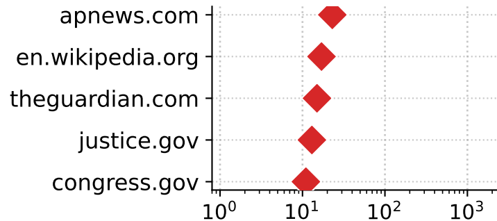
GPT-5-nano
