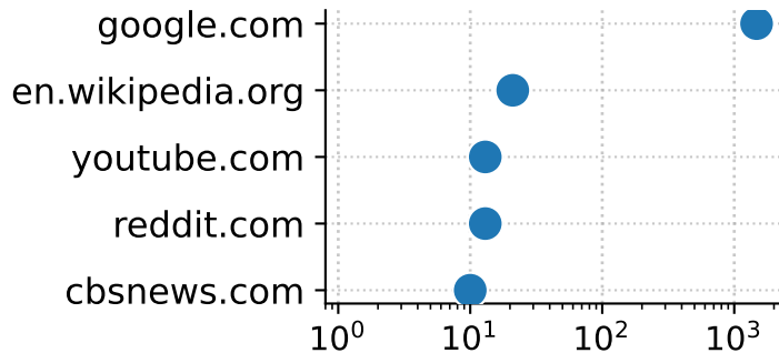
Gemini-2.5-Flash
