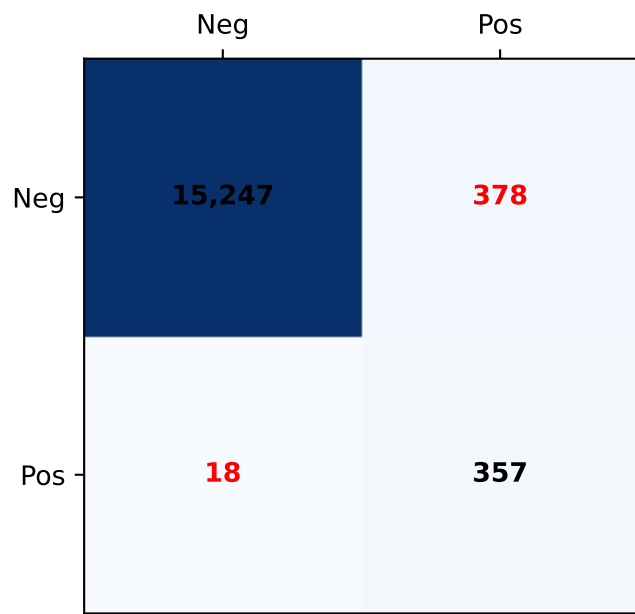
CatBoost
