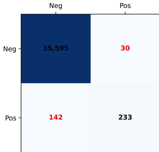
CatBoost
