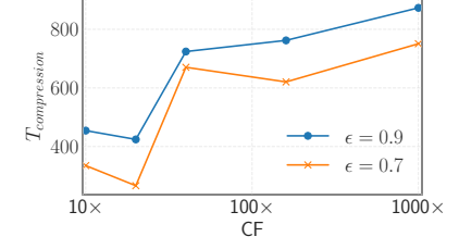
(f) VGG16 T_{compression}
