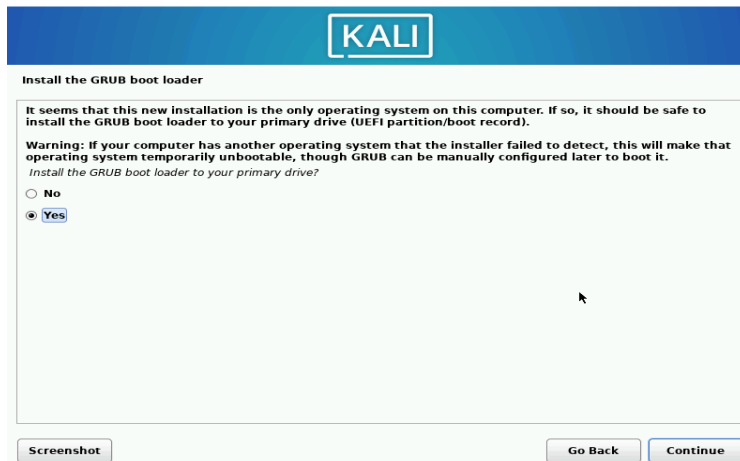
Рисунок 10: Подготовка загрузчика
