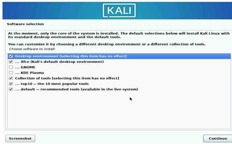
Рисунок 9: Выбор окружения
