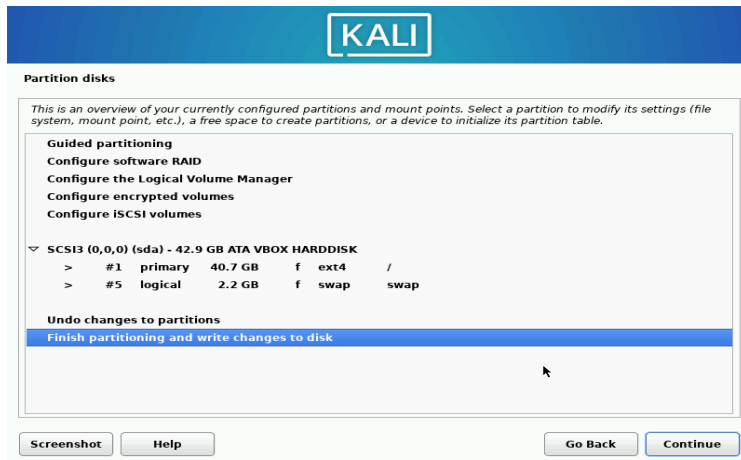
Рисунок 7: Подготовка разделов
