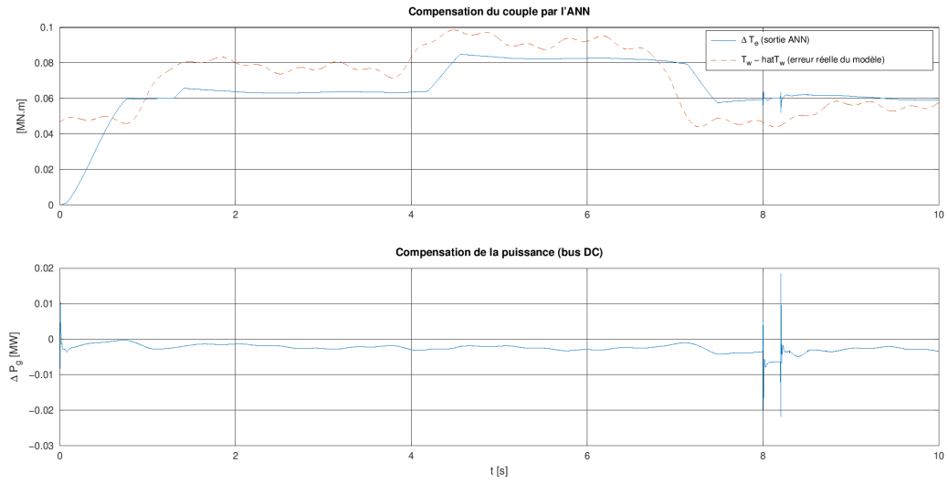
FIGURE 4 – Sortie \Delta T_e de l'ANN comparée à l'erreur réelle du modèle aérodynamique T_w - \hat{T}_w (non connue de l'ANN), et compensation \Delta P_g .
