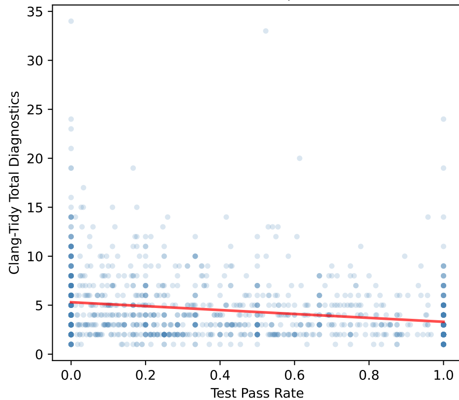
Llama (rho=-0.264, p=1.77e-23)
