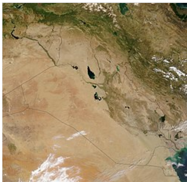
صورة التقطتها وكالة ناسا وتبين خريطة العراق من الفضاء الخارجي
