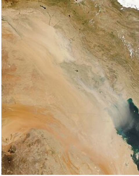
صورة لانساً تظهر عاصفة غبارية تضرب البلاد بتاريخ 30 يوليو عام 2009.
