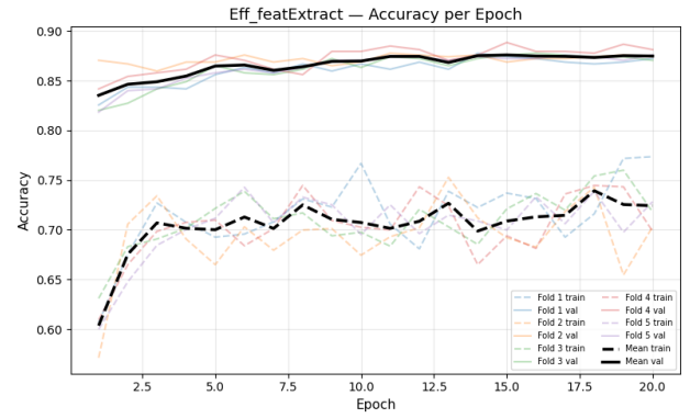
(d) Eff-B3 Feature Extract — Accuracy
