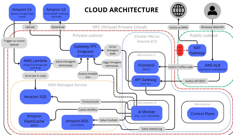
Figura 4: Architettura Cloud su AWS. La VPC isola i nodi worker nelle subnet private, mentre i servizi accessori sono delegati alle offerte fully-managed (S3, SQS, RDS, ElastiCache).
