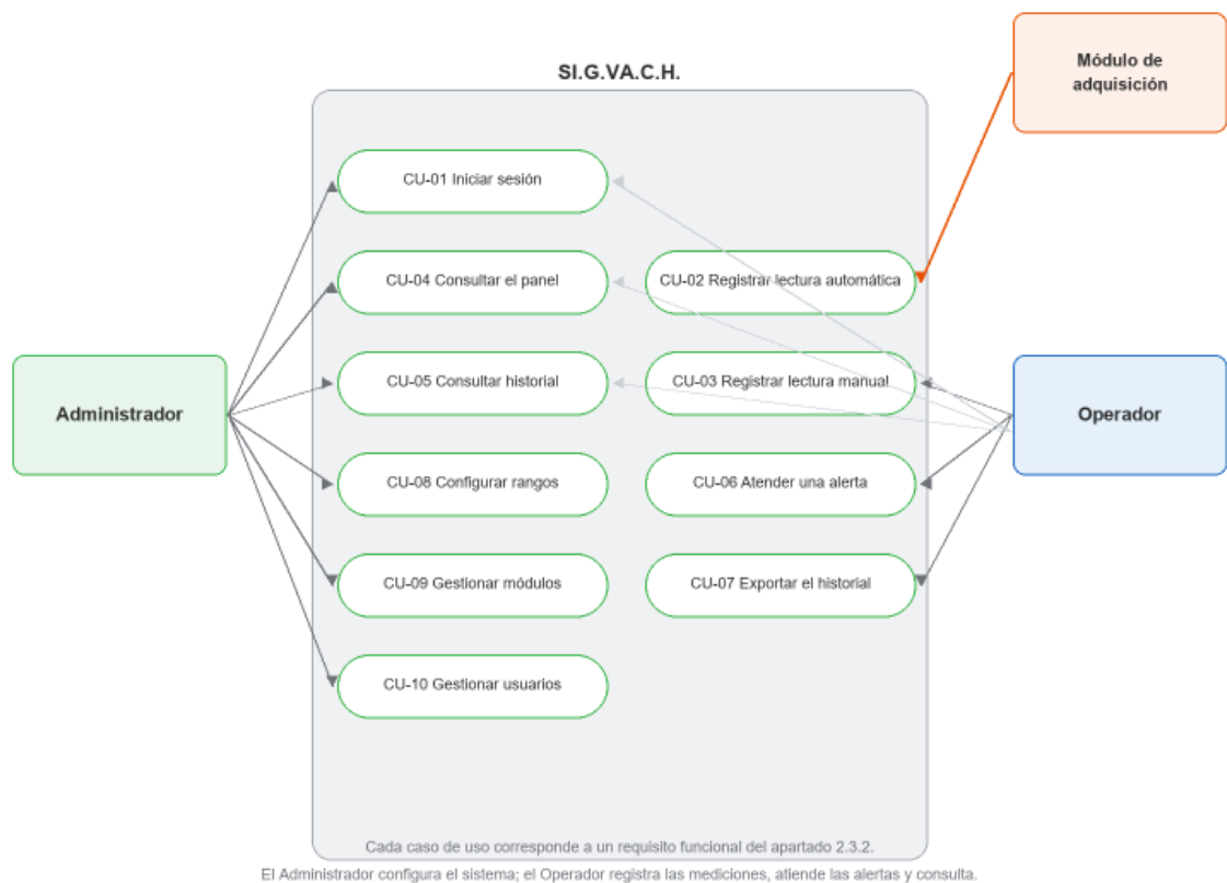
Figura 2. Diagrama de casos de uso del sistema. Fuente: elaboración propia.
