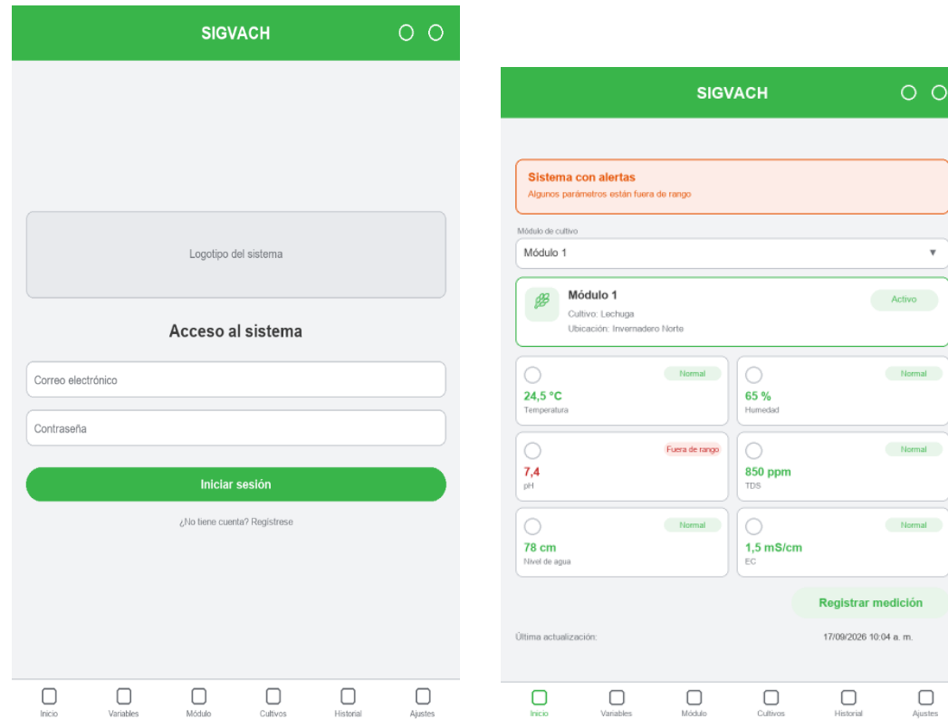
Figura G.3. Wireframes de las pantallas principales. Fuente: elaboración propia.
