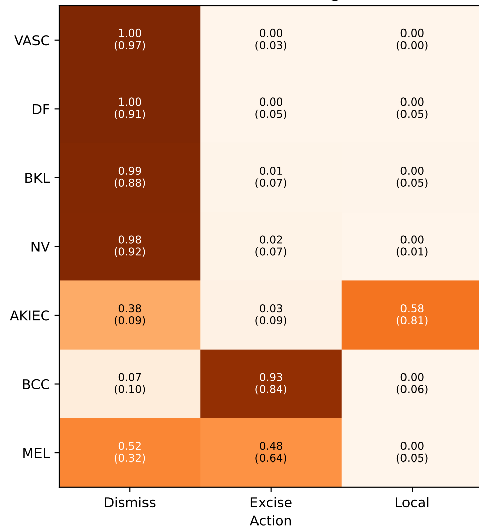
Naive SL (ours / Fig 2f)
