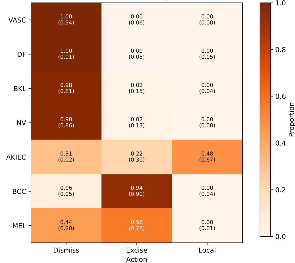
RL DQN (ours / Fig 2h)
