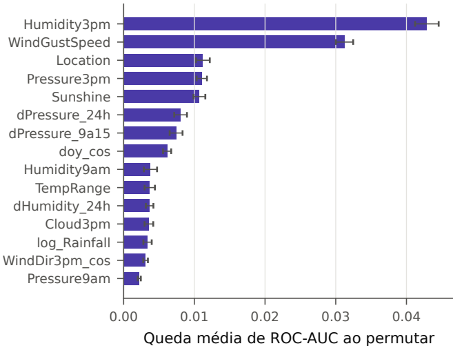
(a) Importância por permutação - LightGBM
