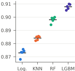
ROC-AUC por dobra
