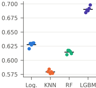
F1 por dobra (limiar 0,5)
