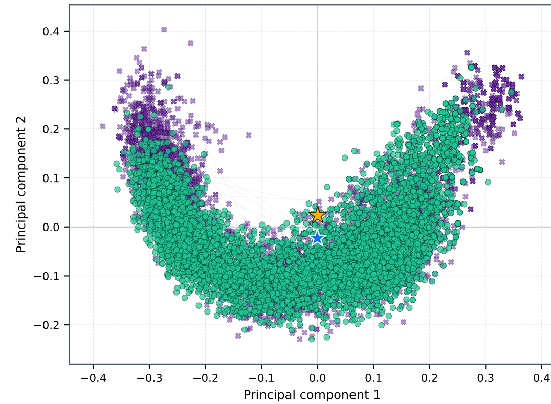
test-dpo (n=6357)
