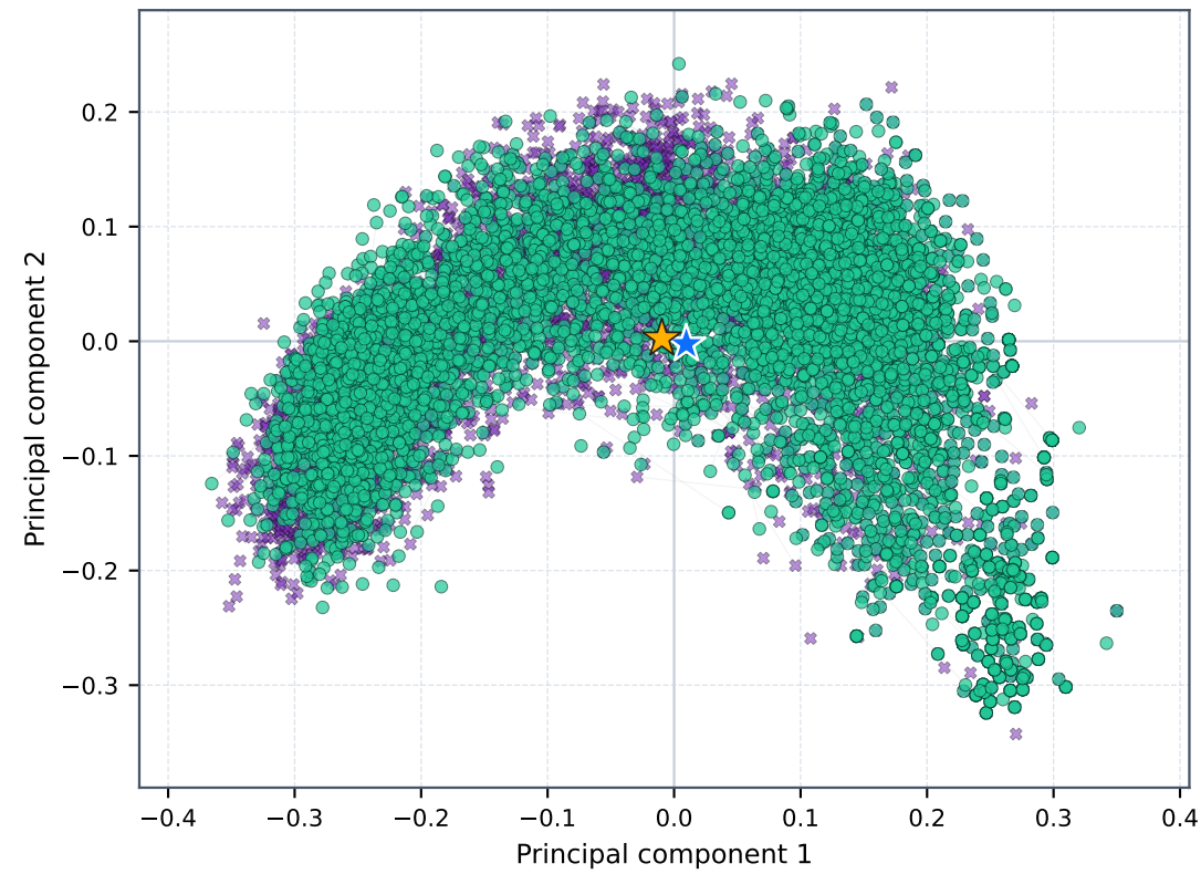
test-sft (n=6357)
