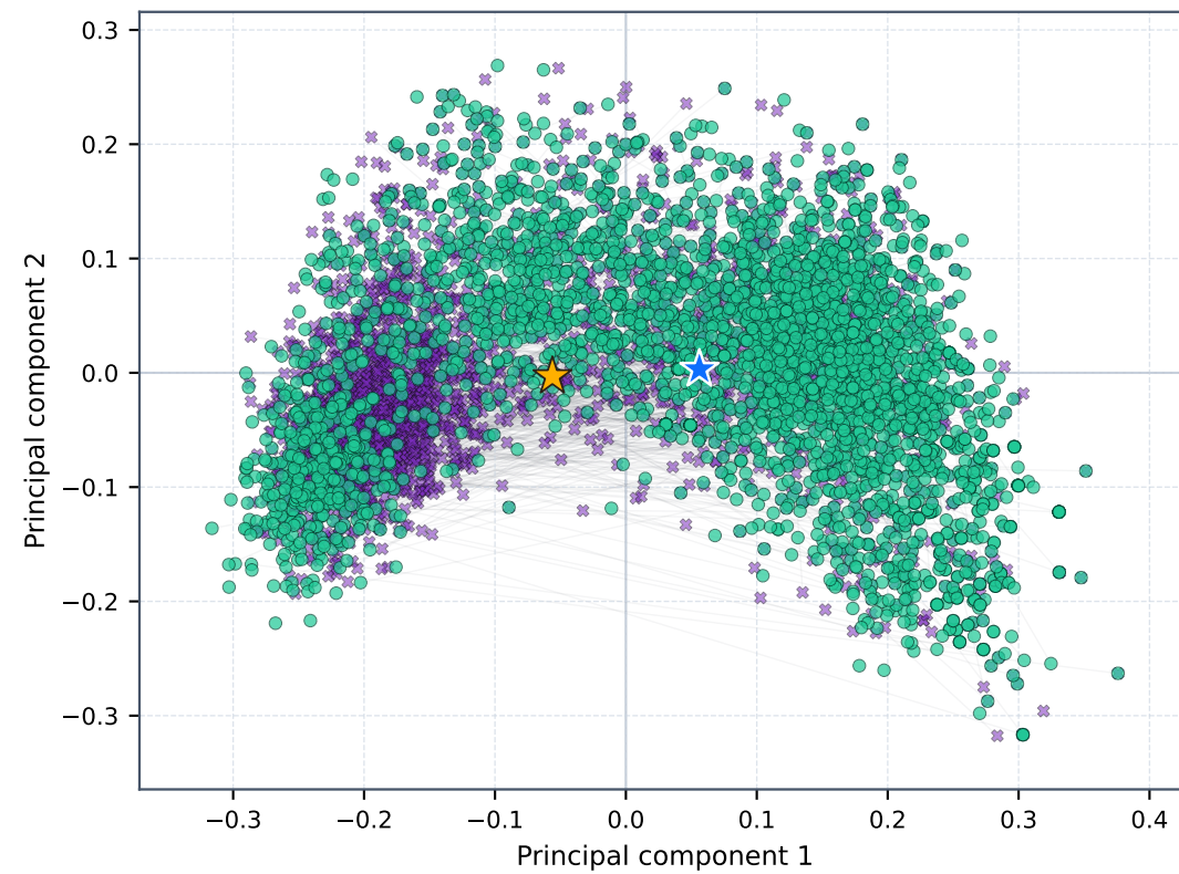
test-hdpo (n=3260)
