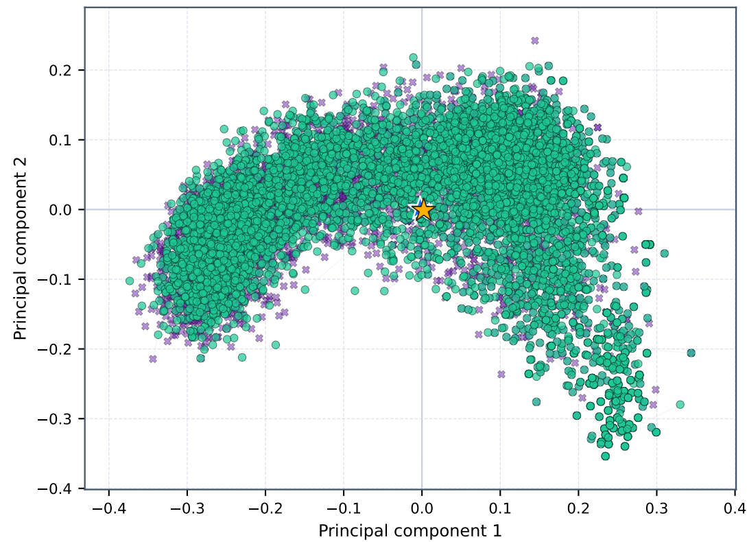
test-bucket-sft (n=6357)
