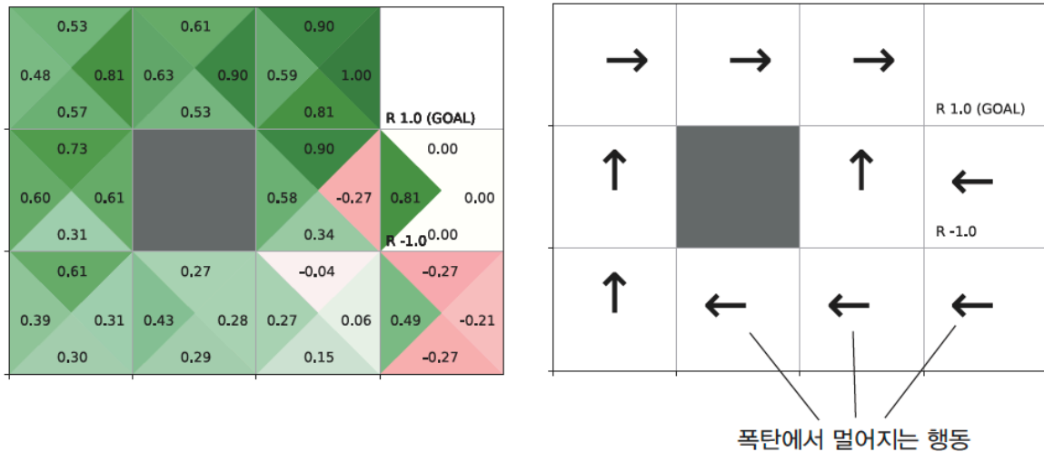
그림 7. 10,000 에피소드로 학습한 Q 함수(왼쪽)와 그것을 탐욕화한 정책(오른쪽). 원서는 아래 줄의 왼쪽 화살표 셋에 “폭탄에서 멀어지는 행동”이라 적어 두었다. 셋 가운데 오른쪽 끝 (2,3)의 LEFT는 최적 정책과 같지만 (2,1)과 (2,2)는 다르며, 그 두 칸이 왜 그렇게 되는지는 아래 본문과 이 절 끝의 [보충]에서 다룬다. 출처: 원서 그림 6-7.
