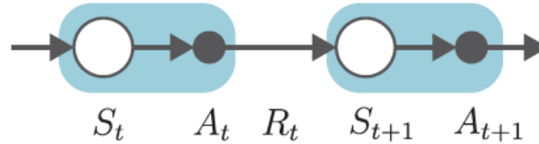
그림 6. 갱신에 필요한 것을 시간 순으로 늘어놓은 것. S_t, A_t, R_t, S_{t+1}, A_{t+1} 다섯이며, 머리글자를 따서 SARSA라 부른다. 오른쪽 끝의 A_{t+1} 까지 정해져야 갱신할 수 있으므로 갱신이 한 걸음 늦게 일어난다. 출처: 원서 그림 6-6.
