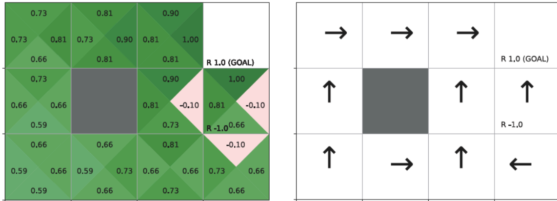
그림 13. Q 러닝의 결과. Q 값이 1.00, 0.90, 0.81, 0.73, 0.66처럼 \gamma 의 거듭제곱으로 정확히 찍히고, 폭탄으로 향하는 행동만 -0.10 = -1 + \gamma \cdot 1.00 이다. 오른쪽 정책은 4장의 최적 정책과 같다. 출처: 원서 그림 6-15.
