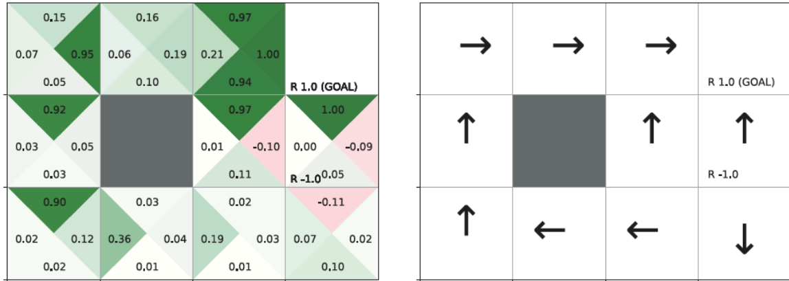
그림 9. 오프-정책 SARSA의 결과. 그림 7와 견주면 폭탄 칸 (1,3)이 UP으로 목표를 향하고 Q 값도 전반적으로 크다. 평가 대상이 해매지 않는 탐욕 정책이라 실수로 폭탄에 빠지는 몫을 셈하지 않기 때문이다. 출처: 원서 그림 6-9.
