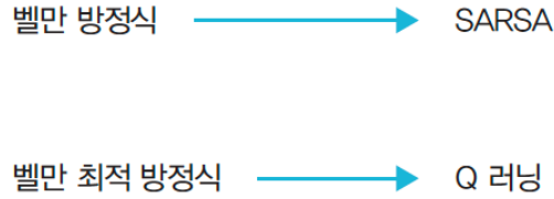
그림 6-10 벨만 방정식과 SARSA, 벨만 최적 방정식과 Q 러닝의 관계
