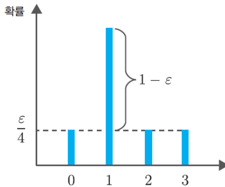
그림 10. \epsilon -탐욕 정책이 각 행동에 주는 확률. 막대 네 개가 모두 \epsilon/4 이상이고, 최선의 행동만 거기서 1 - \epsilon 만큼 더 높다. 확률이 0인 행동이 없으므로 모든 (상태, 행동) 쌍이 언젠가는 시도된다. 출처: 원서 그림 5-15.
