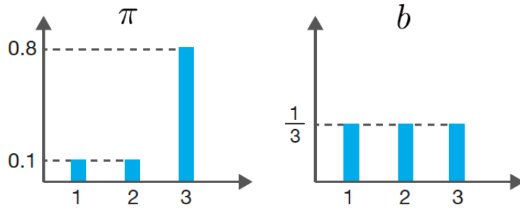
그림 5-19 확률 분포 \pi 와 b
