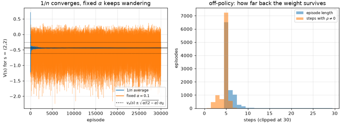
그림 18. 왼쪽: 상태 (2, 2)의 추정치가 에피소드에 따라 움직이는 모습을 시드 여섯 개씩 겹쳐 그린 것. 파란 선( 1/n )은 참값(가로 실선)으로 모여 붙고 주황 선( \alpha = 0.1 )은 점선으로 표시한 \pm\sqrt{\alpha/(2-\alpha)}\sigma_G 의 띠 안에서 끝까지 서성인다. 오른쪽: 오프-정책 예제에서 에피소드 길이와 중요도 가중치가 살아 있는 꼬리 길이의 분포. 부록 A.5에서 다룬다. ch05/paper/fig_mc.py 에서 생성.
