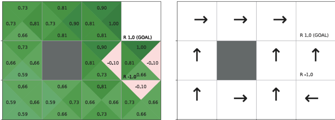
그림 15. Q 러닝의 결과. Q 값이 1.00, 0.90, 0.81, 0.73, 0.66처럼 \gamma 의 거듭제곱으로 정확히 찍히고, 폭탄으로 향하는 행동만 -0.10 = -1 + \gamma \cdot 1.00 이다. 오른쪽 정책은 앞 장의 최적 정책과 같다. 출처: 원서 그림 6-15.
