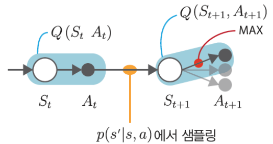
그림 6-14 샘플링 버전 벨만 최적 방정식의 백업 다이어그램
