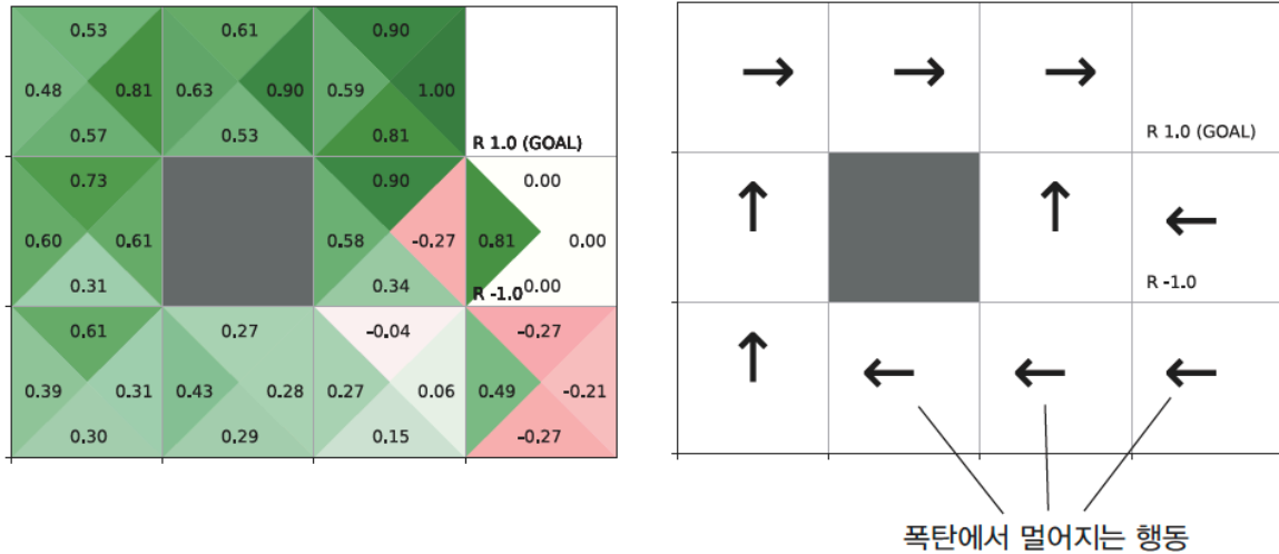
그림 8. 10,000 에피소드로 학습한 Q 함수(왼쪽)와 그것을 탐욕화한 정책(오른쪽). 원서는 아래 줄의 왼쪽 화살표 셋에 “폭탄에서 멀어지는 행동”이라 적어 두었다. 셋 가운데 오른쪽 끝 (2,3)의 LEFT는 최적 정책과 같지만 (2,1)과 (2,2)는 다르며, 그 두 칸이 왜 그렇게 되는지는 이 절 끝의 [보충]에서 다룬다. 출처: 원서 그림 6-7.
