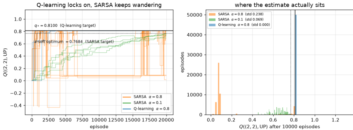
그림 9. 왼쪽: Q((2, 2), \text{UP}) 이 학습 중에 움직이는 모습을 시드 다섯 개씩 겹쳐 그린 것. 파란 선(Q 러닝)은 q_* = 0.8100 에 붙은 뒤 떨어지지 않고, 주황 선(SARSA \alpha = 0.8 )은 위아래로 1이 넘는 폭을 오간다. 초록 선( \alpha = 0.1 )은 느리지만 점선으로 표시한 자기 목표 0.7684를 향해 올라간다. 오른쪽: 10,000 에피소드 이후 그 값이 실제로 머무는 자리의 분포. Q 러닝은 0.8100 한 점에 못 박혀 막대가 하나뿐이다. ch06/paper/fig_td.py에서 생성.
