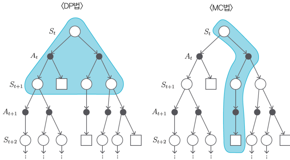
그림 1. DP법(왼쪽)과 MC법(오른쪽)이 쓰는 범위. 왼쪽은 폭이 넓고 깊이가 한 층이다. 다음 상태를 빠짐없이 훑되 한 걸음만 내려가며, 전부 훑으려면 p 와 \pi 를 알아야 한다. 오른쪽은 폭이 한 줄기고 깊이가 끝까지다. 모델은 필요 없지만 바닥에 닿아야, 곧 에피소드가 끝나야 값이 나온다. 출처: 원서 그림 6-1.
