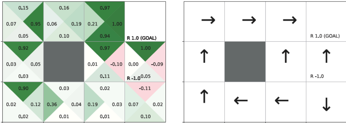
그림 11. 오프-정책 SARSA의 결과. 그림 8와 견주면 폭탄 칸 (1,3)이 UP으로 목표를 향하고 Q 값도 전반적으로 크다. 평가 대상이 헤매지 않는 탐욕 정책이라 실수로 폭탄에 빠지는 몫을 셈하지 않기 때문이다. 출처: 원서 그림 6-9.
