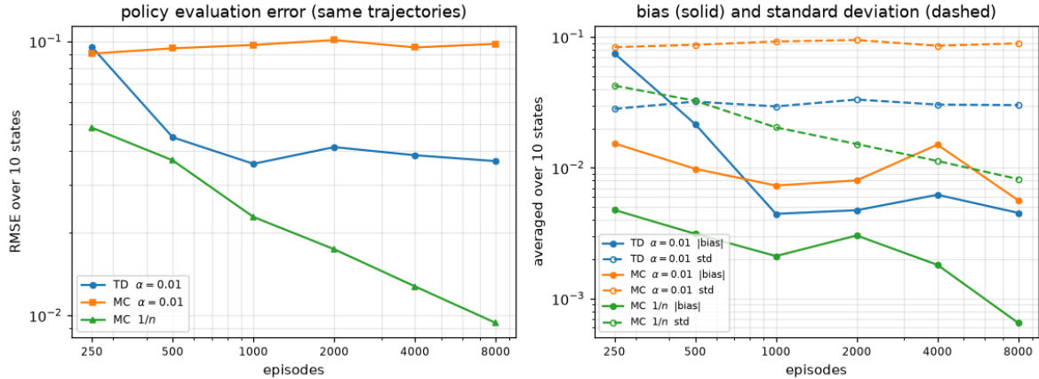
그림 6. 왼쪽: 세 방법의 RMSE. 고정값 \alpha 를 쓰는 두 방법은 일찍 바닥에 닿아 더 내려가지 않고 1/n 평균만 계속 내려간다. 오른쪽: 같은 실험을 편향(실선)과 표준편차(점선)로 나눈 것. TD법의 파란 실선이 250 에피소드에서 가장 높은 자리에서 시작해 가파르게 떨어지는 것이 부트스트래핑의 편향이 걸히는 모습이고, 파란 점선이 주황 점선의 3분의 1 자리에 가로놓인 것이 분산의 차이이다. ch06/paper/fig_td.py에서 생성.
