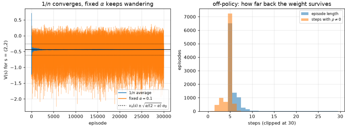
그림 15. 왼쪽: 상태 (2, 2)의 추정치가 에피소드에 따라 움직이는 모습을 시드 여섯 개씩 겹쳐 그린 것. 파란 선( 1/n )은 참값(가로 실선)으로 모여 붙고 주황 선( \alpha = 0.1 )은 점선으로 표시한 \pm \sqrt{\alpha/(2-\alpha)} \sigma_G 의 띠 안에서 끝까지 서성인다. 오른쪽: 오프-정책 예제에서 에피소드 길이와 중요도 가중치가 살아 있는 꼬리 길이의 분포. §5.5 끝의 [보충]에서 다룬다. ch05/paper/fig_mc.py에서 생성.
