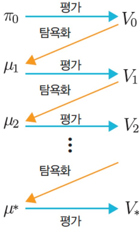
그림 12. 정책 반복법. 파란 화살표(평가)와 주황 화살표(탐욕화)가 번갈아 이어지며 내려간다. \pi_0 \rightarrow V_0 \rightarrow \mu_1 \rightarrow V_1 \rightarrow \mu_2 \rightarrow \cdots \rightarrow \mu_* \rightarrow V_* . 출처: 원서 그림 4-14.
